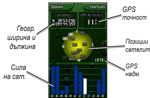
Страница Сателити
