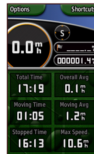
Автомобилен режим
