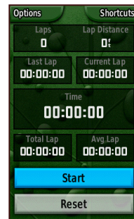
Стр.секундомер
