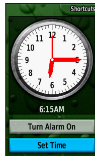
Стр.настройка аларма
