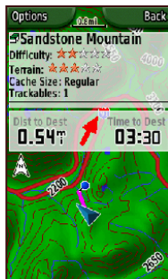
Стран. геокеш
