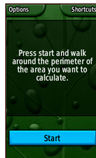
Стр.старт измерване
