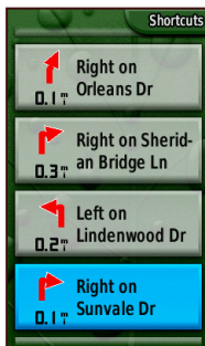
Акт.маршрут завой-по-завой
