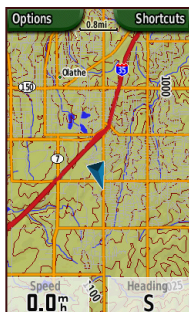
Страница карта
